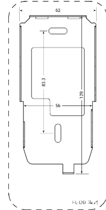
드릴링 템플릿
